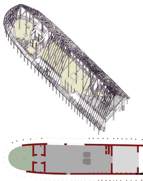
Fig. 4. L'Edificio di Lefkandi. Da MALACRINO 2010.
